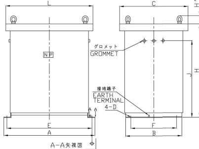
図-3 ・TTSB-6KLWC~TTSB-100KLG
